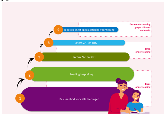
Figuur 5.4 Cascademodel
